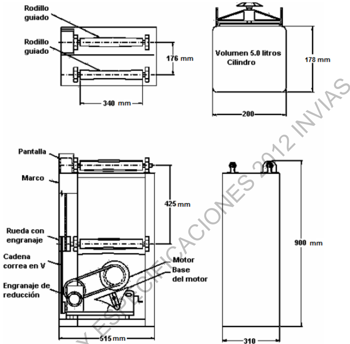
Figura 238 - 2. Aparato Micro-Deval
